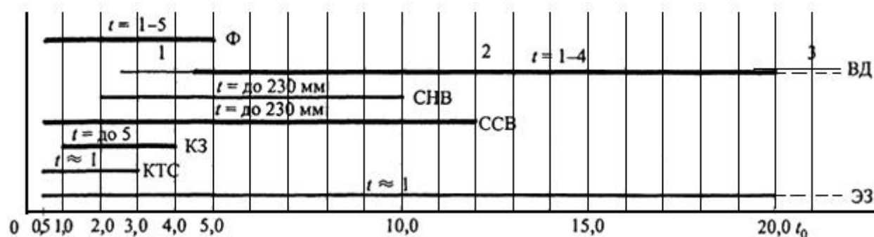
4.2 - Область применения различных видов СМС в зависимости от сочетания толщин соединяемых элементов
