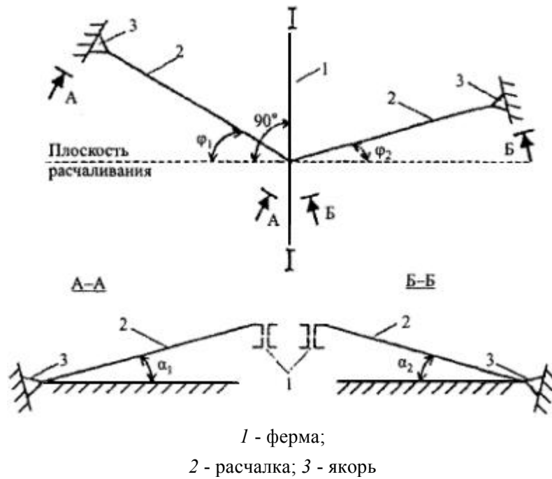
Рисунок К.2 - Схема раскрепления ферм расчалками
