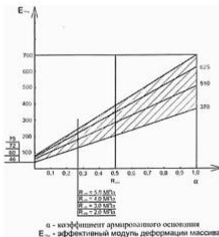
Рисунок Ф.1 - График зависимости эффективного модуля деформации армированного ГЦЭ
