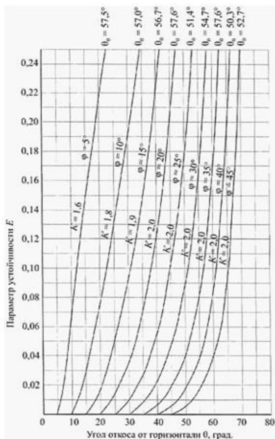
Рисунок В.3 - Графики для определения крутизны откоса при 1 < K < 2 (в ред. Изменения № 3 , утв. Приказом Минстроя РФ от 16.12.2021 N 954/пр)
