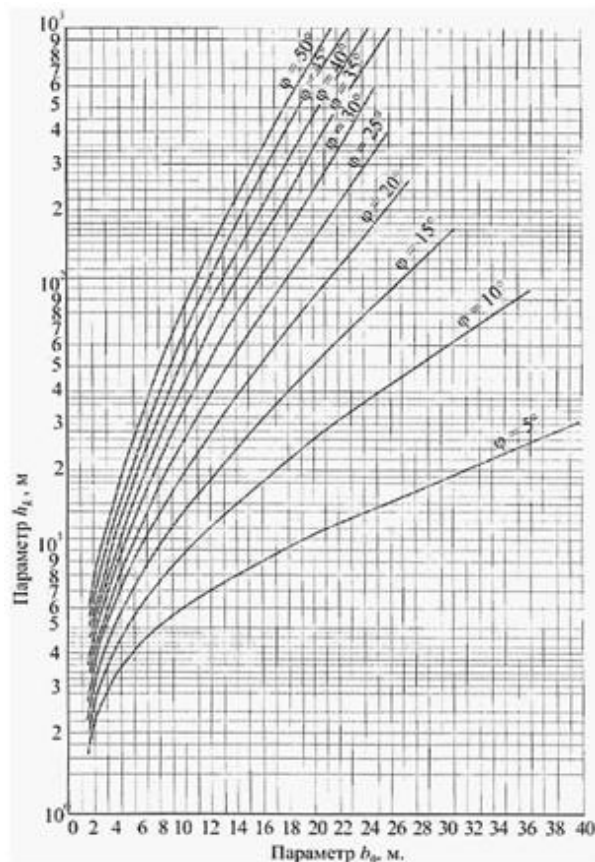
Рисунок В.6 - Графики для определения параметра b_0
