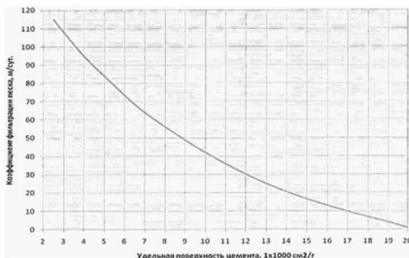
Рисунок Т.1 - График зависимости проникающей способности цементного раствора от
